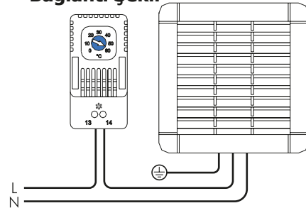
Soğutma Termostatı THV Bağlantı Şekli
