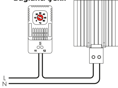
Isıtma Termostatı THR Bağlantı Şekli
