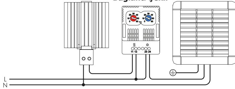
Isıtma - Soğutma Termostatı THRV Bağlantı Şekli
