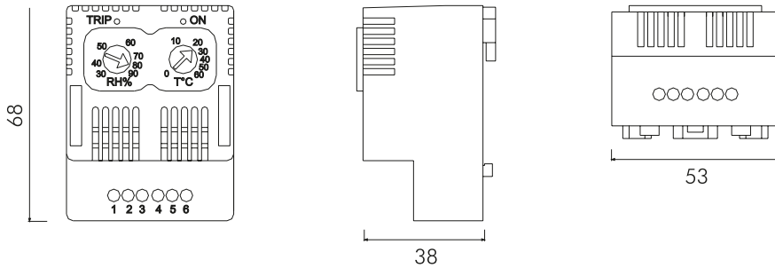
Elektronik Higrostat ETUH 22 Bağlantı Şekli
