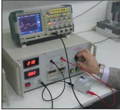
TS EN 61008-1 madde 9.19.1'e göre yapılan gerilim darbelerinin sebep olduğu akım dalgaları durumunda kaçak akım koruma şalterlerinin davranışının doğrulanması (tepe akımı 200 A)
