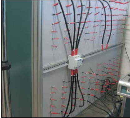
TS EN 61008-1 madde 9.8 'e göre yapılan sıcaklık artışı deneyi.
