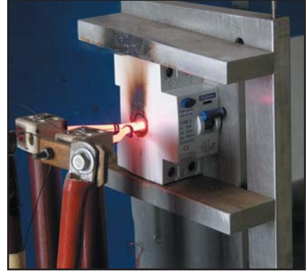
TS EN 61008-1 madde 9.14 'e göre yapılan olağan dışı ısıya ve ateşe dayanıklılık deneyi
